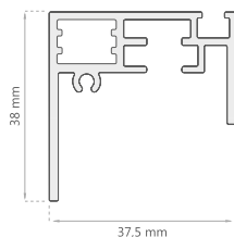
Marco Imán D-2100
