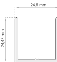
Expansor Marco Fijo Corto J-1110
