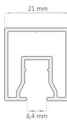
Marco Fijo Corto K-0304/6
