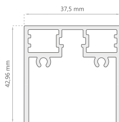
Marco Lateral 2 Hojas Correderas D-2117
