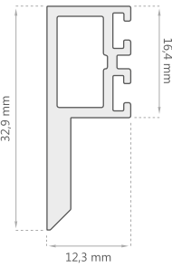
Expansor Marco Fijo Corto J-1110
