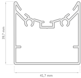
Marco Fijo D-2013
