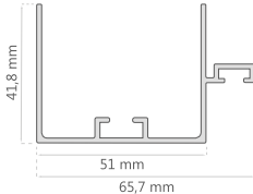
Guía Superior D-2065
