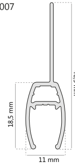
PERFIL HOJA RULETA D-2007
