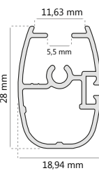
PERFIL FIJO HOJA D-2003
