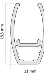
PERFIL FIJO PALITOD-2006
