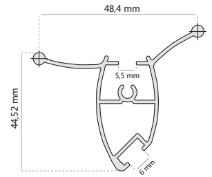
PERFIL TIRADOR ANGULAR D-2008
