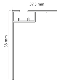
MARCO FIJO D-2002
