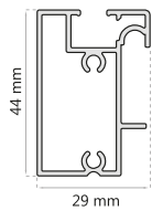
GUÍA D-2053/6
