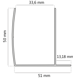
EXPANSOR D-2003
