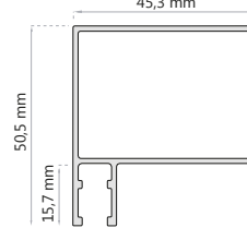
ESQUINERO FIJO LATERAL D-2054
