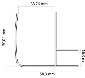
ESQUINERO FIJO LATERAL 100941
