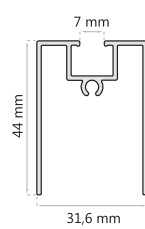
MARCO FIJO D-2056
