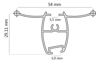
PERFIL TIRADOR FRONTAL /SEMIC. D-2005
